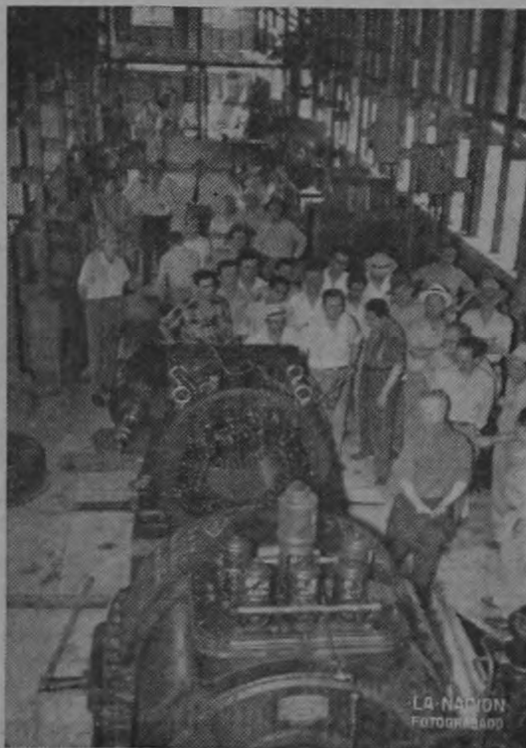
Turbina de vapor y generador eléctrico de 750 K. V. A. Al fondo, el taller mecánico
